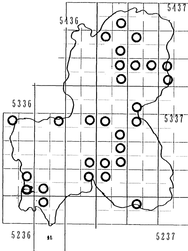
図6 トボシガラ分布図 ( Festuca parvigluma )
