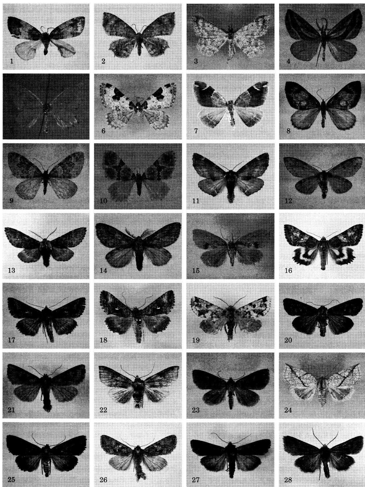
図5. 注目すべき種類Ⅱ. 1:ヒメナカジロトガリバ, 2:ウスチャオビフタオ, 3:ダイセンハグルマエダシャク, 4:ハスオビカバエダシャク, 5:シラユキナミシャク, 6:クロモンミヤマナミシャク, 7:キジマソトグロナミシャク, 8:ネアカナカジロナミシャク, 9:ミヤマクロオビナミシャク, 10:ヤハズナミシャク, 11:コクシエグリシャチホコ, 12:ゴマダラシャチホコ, 13:アマギシャチホコ, 14:ブナアオシャチホコ, 15:オレクギリンガ, 16:アサマキシタバ, 17:ガマキンウワバ, 18:アルプスギンウワバ, 19:ミヤマゴマキリガ, 20:ホソバミドリヨトウ, 21:ミヤマチャイロヨトウ, 22:ツチイロキリガ, 23:フタスジキリガ, 24:キイロトガリヨトウ, 25:クロヨトウ, 26:ムラサキヨトウ, 27:クモマウスグロヤガ, 28:ナカトビヤガ.
