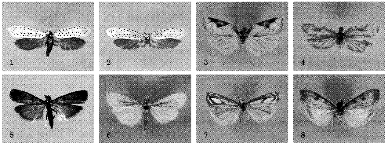
図4. 注目すべき種類 I. 1: サクラスガ, 2: マユミオオスガ, 3: ウツギアミメハマキ, 4: ウスジロハマキ, 5: フタテンアカオビマダラメイガ, 6: ミヤマウスギンツトガ, 7: オオヒシモンツトガ, 8: チャモンノメイガ。
