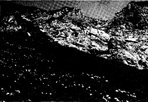
写真13 シナノキンバイ・ハクサンイチゲが目立つ杓子平のお花畑。
