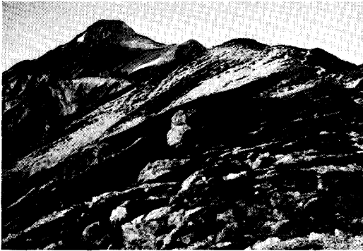
写真9 笠ヶ岳の北尾根、東側斜面。ハイマツは凸地に斑紋状に生育。
