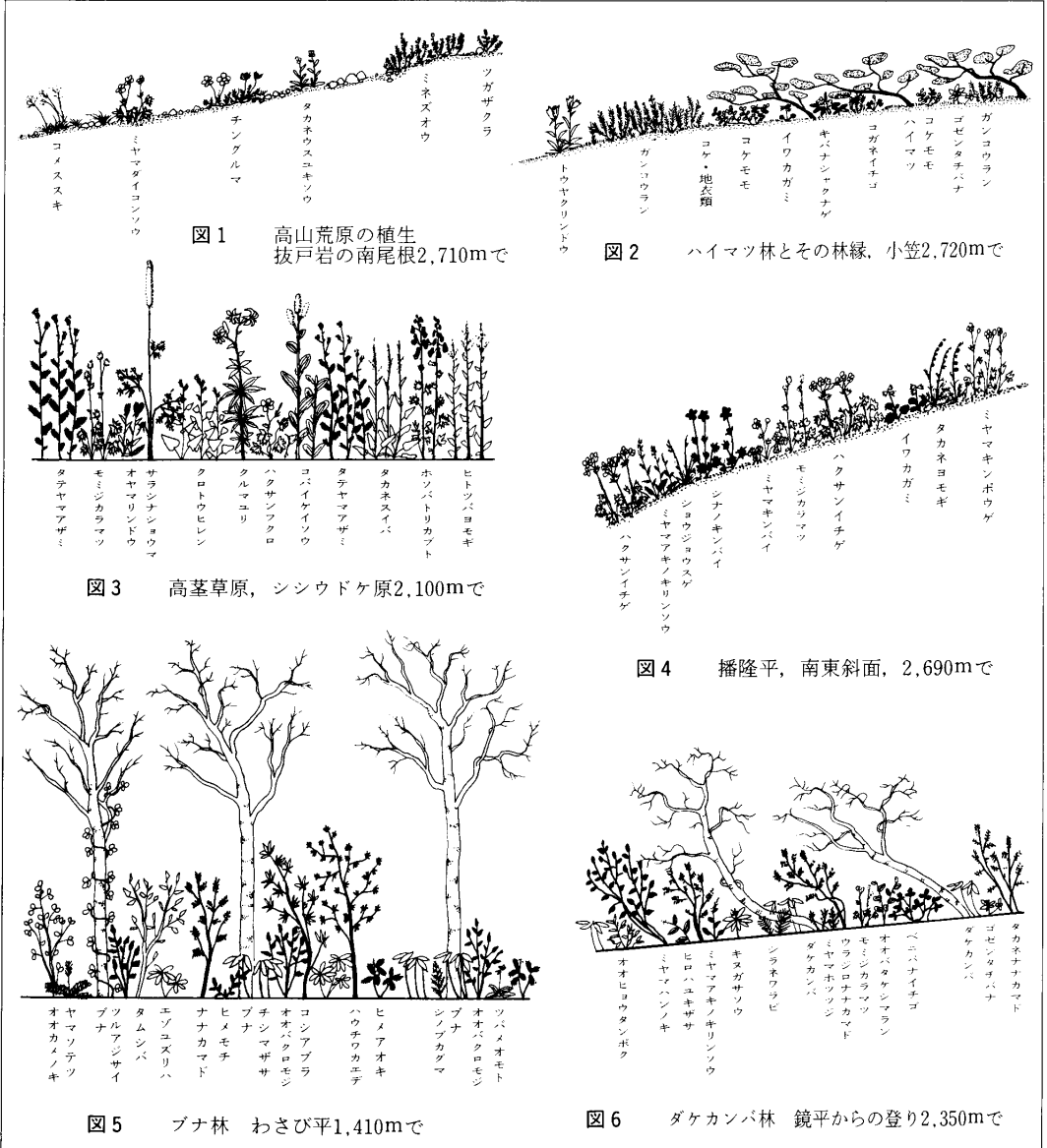
付図 代表的な植生の断面スケッチ
