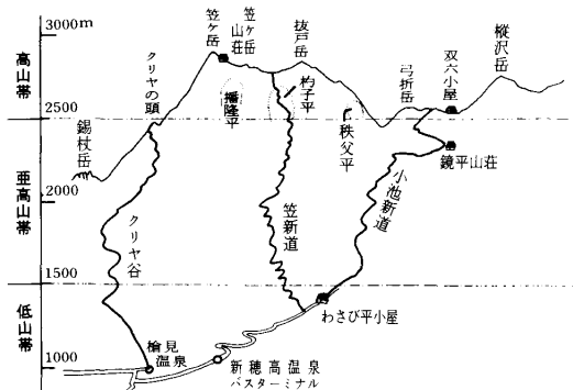
図1 笠ヶ岳連峰の植物垂直分布帯
