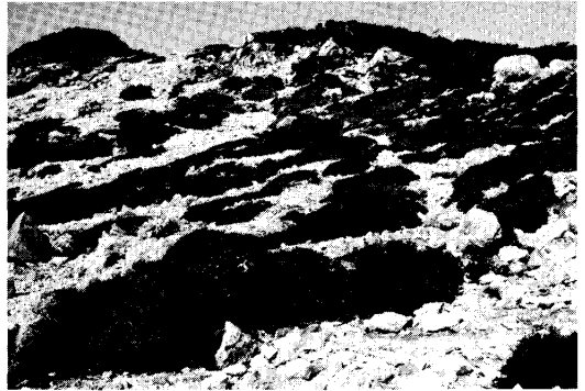
写真10 斑紋状に生育するミネズオウ。チングルマ等の矮生低木群落。同左。
